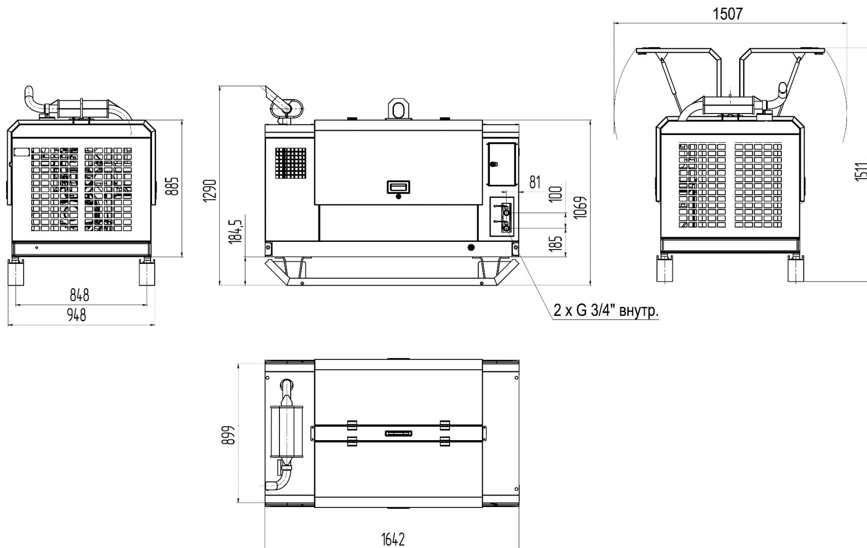
Рисунок 2б – Общий вид станции компрессорной, габаритные и присоединительные размеры.
